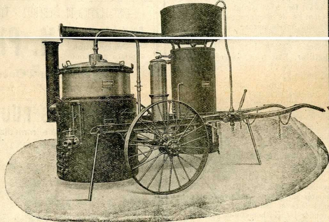
Alambic à feu nu. Degré réglable à volonté. Colonne de concentration syst. Cazagne B. S. G. D. G.
