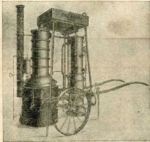
Appareil continu roulant à feu nu
