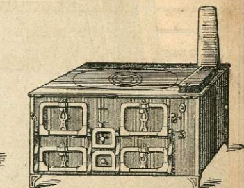
Fourneau à deux fours, deux étuves Réservoir à eau chaude, cendrier trieur
