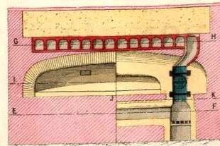
Coupe sur A.B.C.D.
