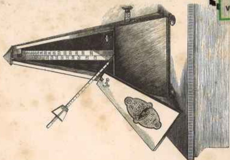
Métromome Magzel à sonnerie, indiquant le premier temps de toutes les mesures 2, 3, 4 et 6/8.
