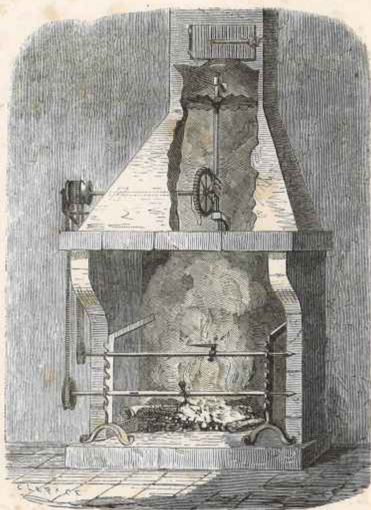
Tournebroche à fumée et ses accessoires.
